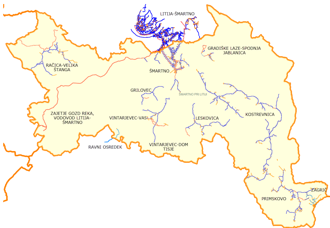
Slika: Prikaz vodovodnih omrežij v občini Šmartno pri Litiji v upravljanju KSP Litija d.o.o.
